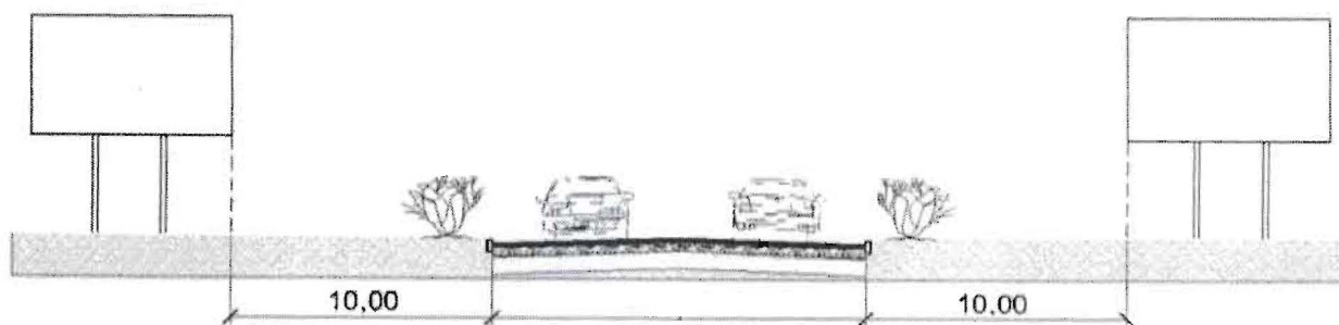
А. Схема размещения рекламных конструкций вне населенного пункта
